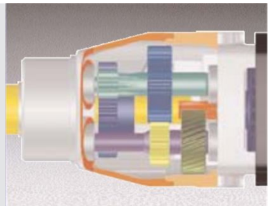
Трёхступенчатый редуктор в корпусе из алюминиевого сплава
